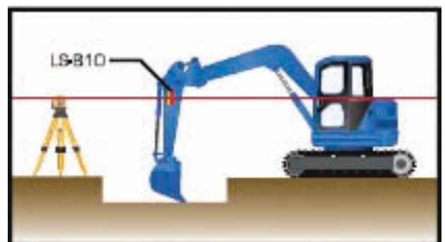
Gebruik als machineontvanger op graafmachine m.b.v. magneetbevestiging
