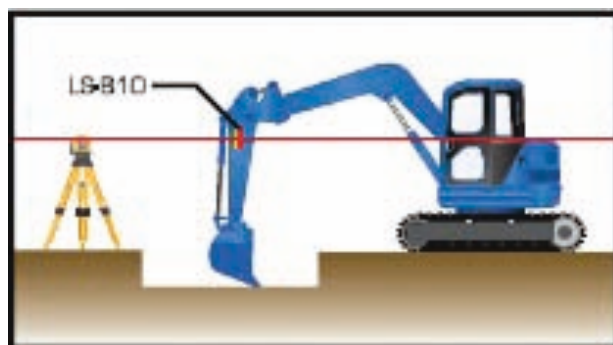
Gebruik als machineontvanger op graafmachine m.b.v. magneetbevestiging
